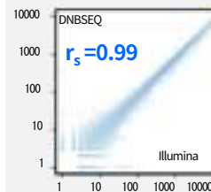
DNBSEQとIlluminaシーケンサーの比較
