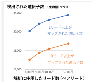
取得リード数と検出遺伝子数の関係
